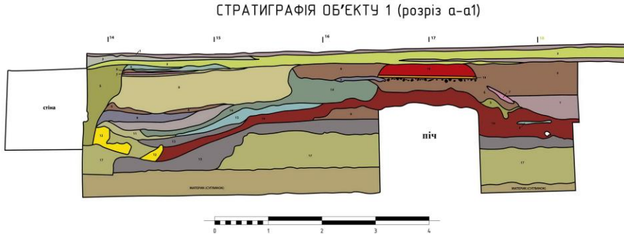
Рис. 5. Розріз об'єкту № 1 по лінії а-а1. Умовні позначення: 1 – мішаний гумусований шар; 2 – чорноземний ґрунт темного кольору; 3 – будівельне сміття II половини XX століття; 4 – горілий шар коричневого ґрунту з вуглинками; 5 – викид ґрунту з-під траншеї під стіну, або при будівництві підвалу з матеріалами XIX ст.; 6 – суглинок; 7 – сірий шар ґрунту, мішаний; 8 – сірий шар ґрунту з вкрапленнями вуглинок, дрібного каміння, обмазки та фрагментів будівельної кераміки і керамічного посуду II половини XVII ст.; 9 – стерильний шар ґрунту сірого кольору; 10 – ґрунт темного кольору з вуглинками та частинами обмазки; 11 – скупчення обмазки; 12 – глиняні "вальки"; 13 – щільний гумусований шар темного кольору з включеннями вуглинок, кісток, кераміки 2 половини XIII–XIV ст.; 14 – шар глини з вкрапленнями обмазки; 15 – шар ґрунту сірого кольору з мілким камінням; 16 – шар сірого ґрунту з обмазкою; 17 – шар суглинку бурого кольору з матеріалами трипільської культури; 18 – печина; 19 – долівка печі
